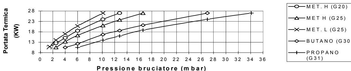
2.11.1 DIAGRAMMA PRESSIONE GAS - PORTATA TERMICA
