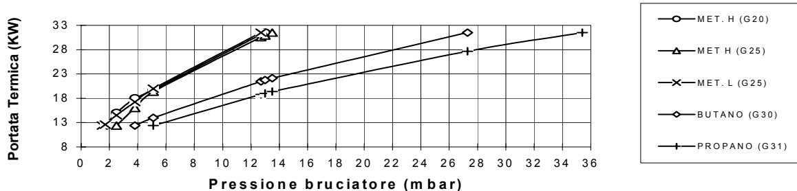
2.12.1 DIAGRAMMA PRESSIONE GAS - PORTATA TERMICA
