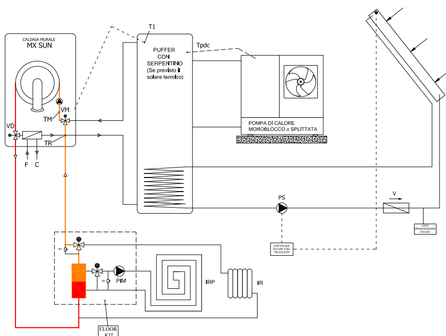
Schema con caldaia spenta o accesa e integrazione con fonti rinnovabili attive
